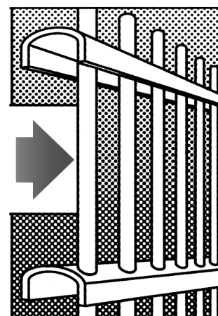
U-Profil / Profil U 9/20/9/2 mm Rundstäbe / Tiges rondes Ø 6 mm
