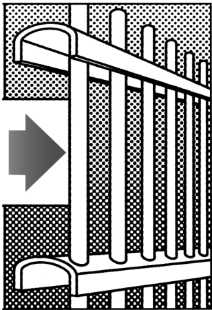
U-Profil / Profil U 9/20/9/2 mm Rundstäbe / Tiges rondes Ø 6 mm
